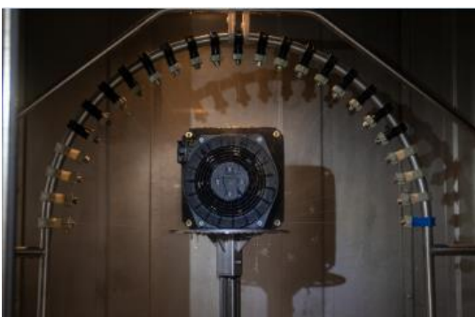
Bild 3: In der IP-Prüfkammer werden Elektroniken und Ventilatoren standardisierten Schutzart-Tests gemäß IP-Code gegen Eindringen von Feuchtigkeit unterzogen.
